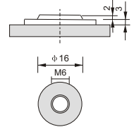
Anschluss T6
